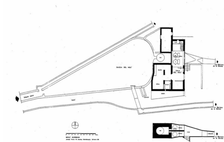
Planta d'un molí hidràulic
